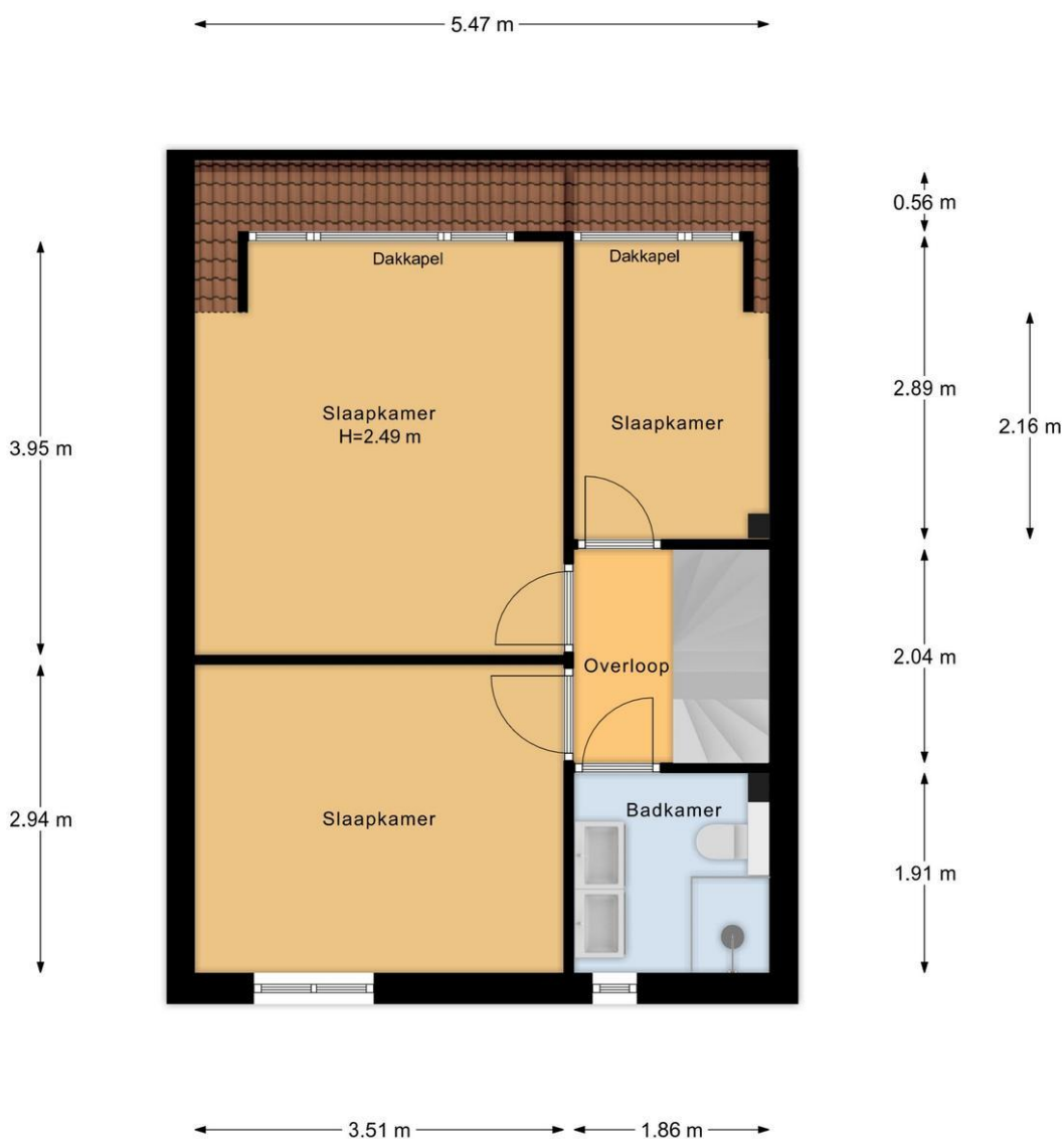
1e Verdieping
