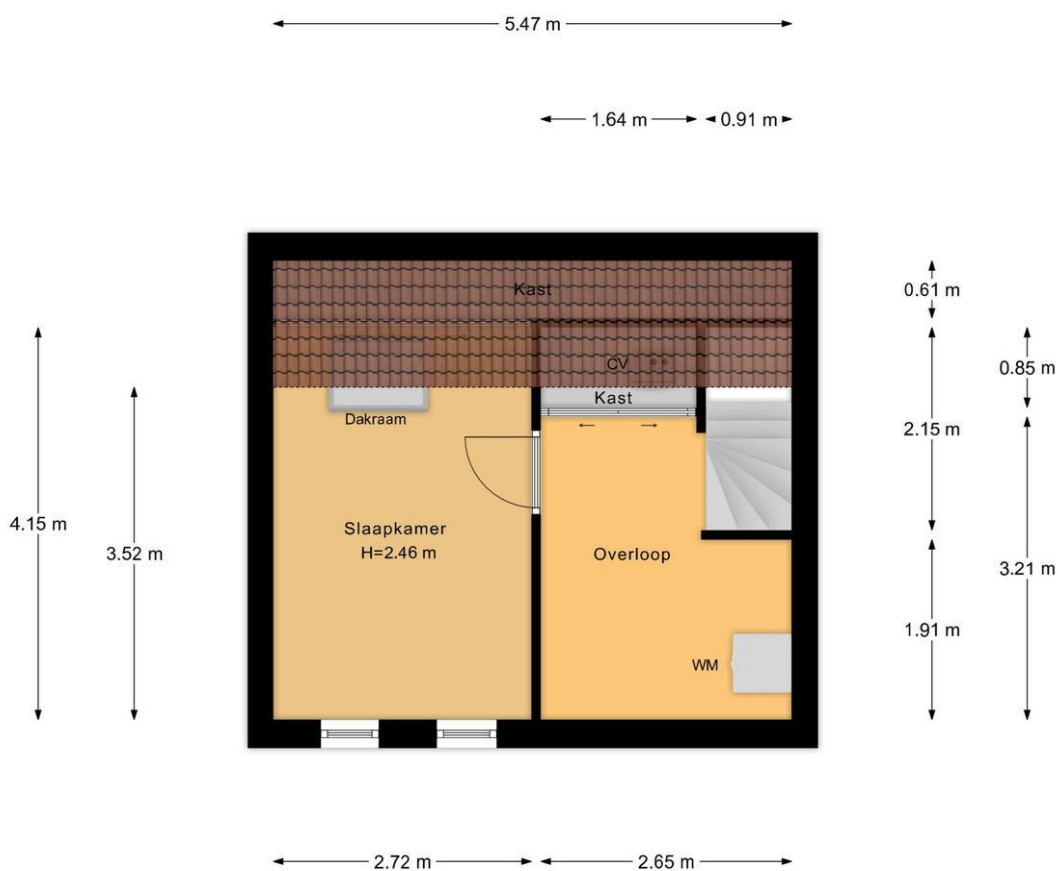
2e Verdieping
