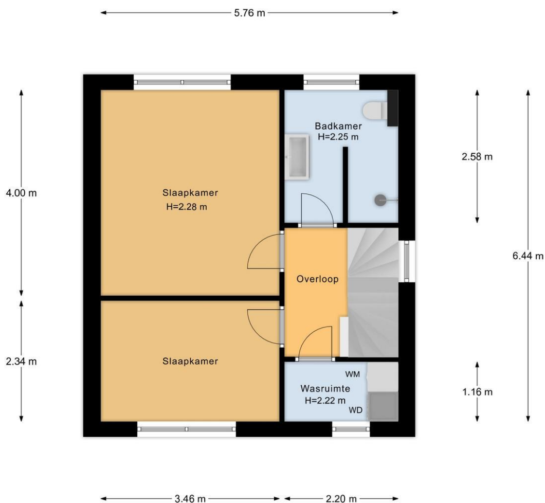
Eerste Verdieping
